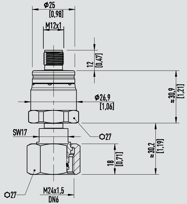
Connettore circolare M12 x 1, versione in plastica, adattatore DN 6
