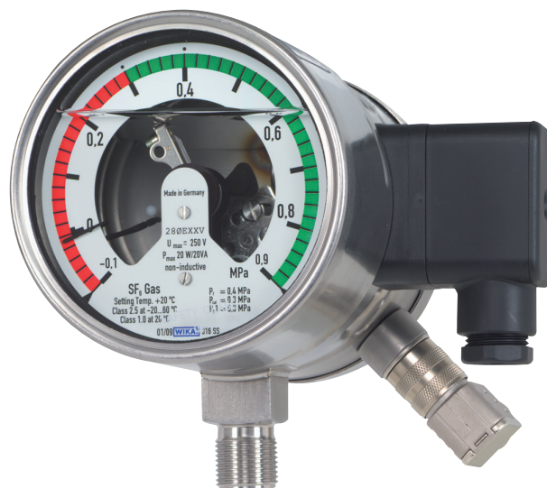
Монитор плотности газа со встроенным преобразователем, модель GDM-100-TI
