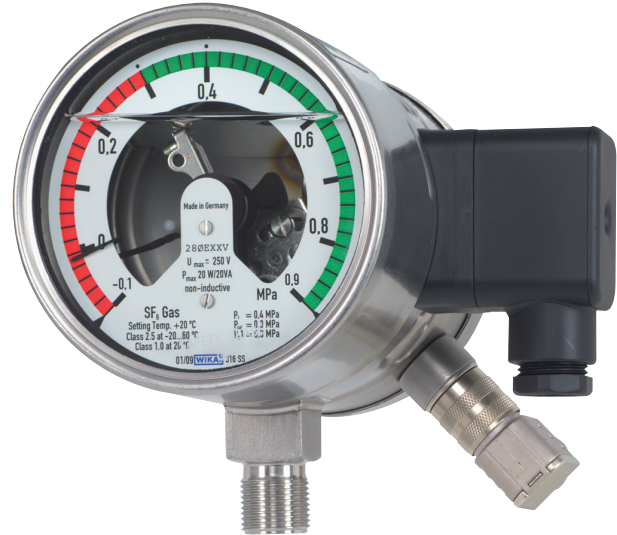
Monitor de densidade de gás com transmissor integrado, modelo GDM-100-TI
